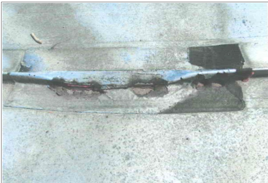
Fotografia obrazująca uszkodzenie uszczelnienia pokrycia.
