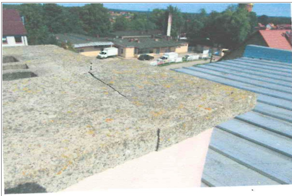
Fotografia obrazująca uszkodzoną czapkę na kominie.
