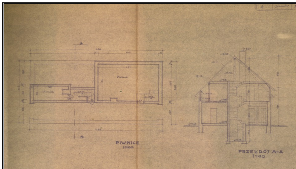
Rzut piwnic
