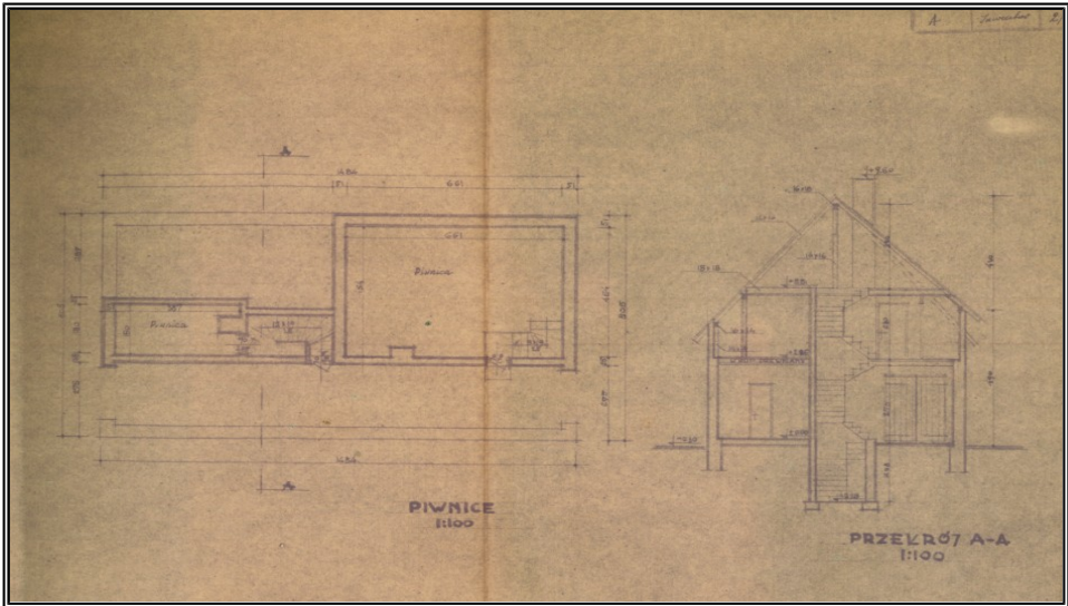
Rzut piwnic
