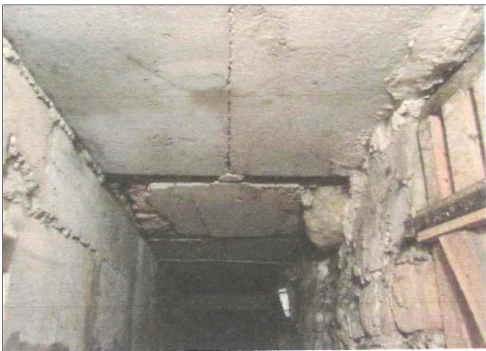
Fotografia obrazująca fragment stropu płytowego na belkach stalowych
